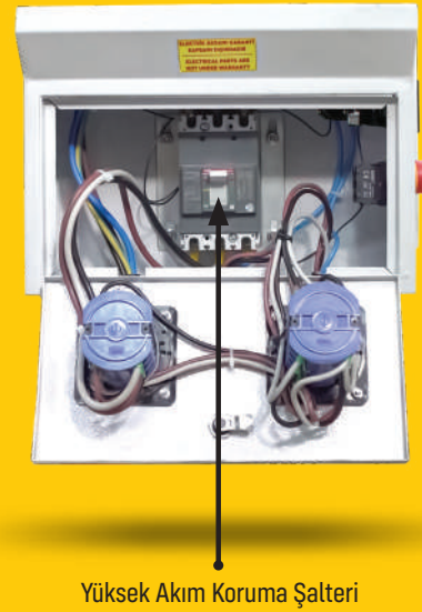
Elektrik Kontrol Panosu (Kapak açık pozisyonu)
