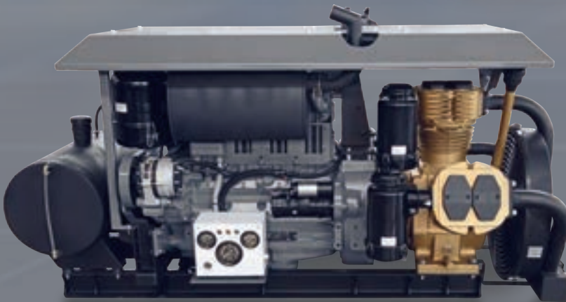
G160-3 NEW DIESEL ENGINE کمپرسور 3 راس مع ماکینه جدیدہ
