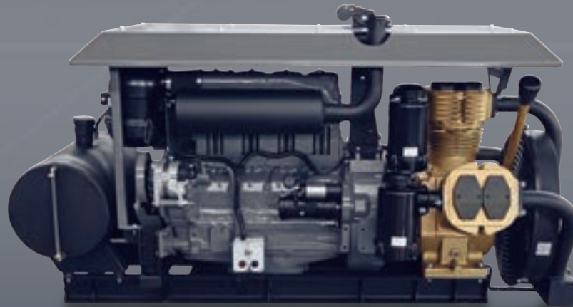
G160-3 RE-NEWED DIESEL ENGINE کمپرسور 3 راس مع ماکینه مجددہ
